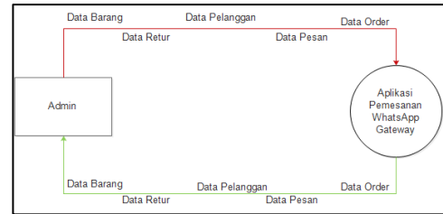
Gambar 5. Diagram Konteks
