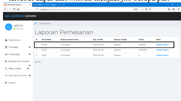
Gambar 19. Menu Laporan.
