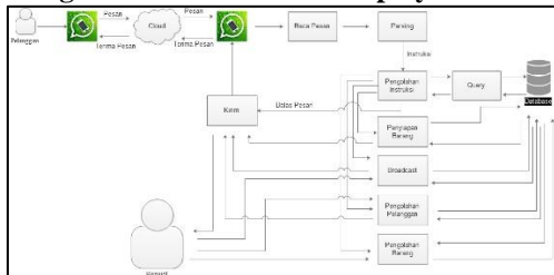
Gambar 3. Arsitektur Deployment.
